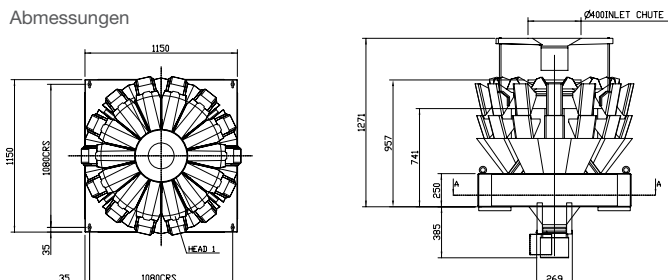
Abmessungen
