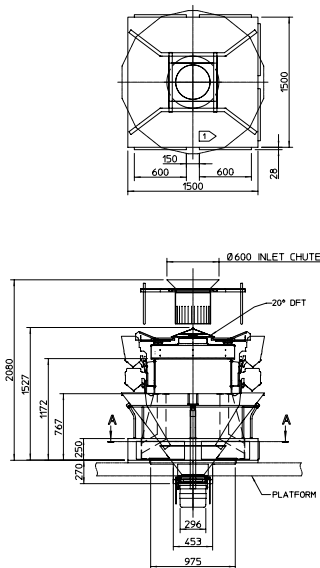
Abmessungen
