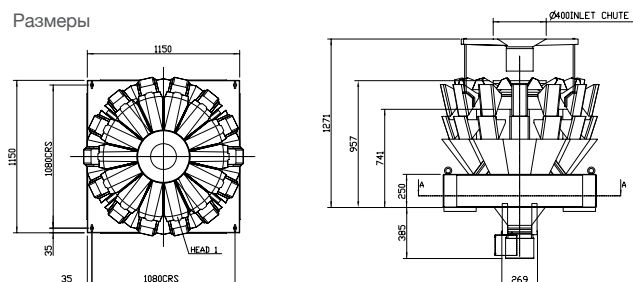
Размеры
