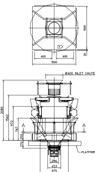
Abmessungen
