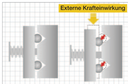
Die Funktion DFL (Dislocating Force Limiter) schützt die Wägezelle gegen externe Störeinflüsse. Das bedeutet weniger Reparaturen und Ersatzteile sowie maximale Verfügbarkeit.
